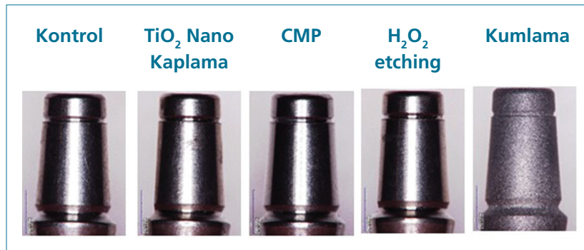
Resim 1: Kontrol ve deney gruplarının temas açısı ölçümleri.
